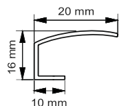
Prowadnica standardowa
