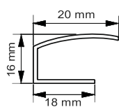
Prowadnica szeroka
