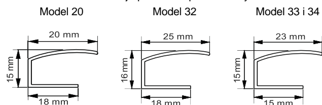
Przekroje prowadnic przestrzennych
